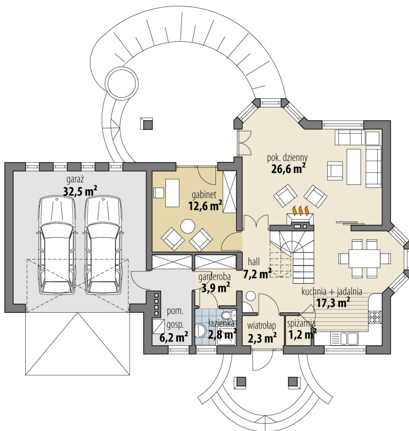
RZUT PARTER
