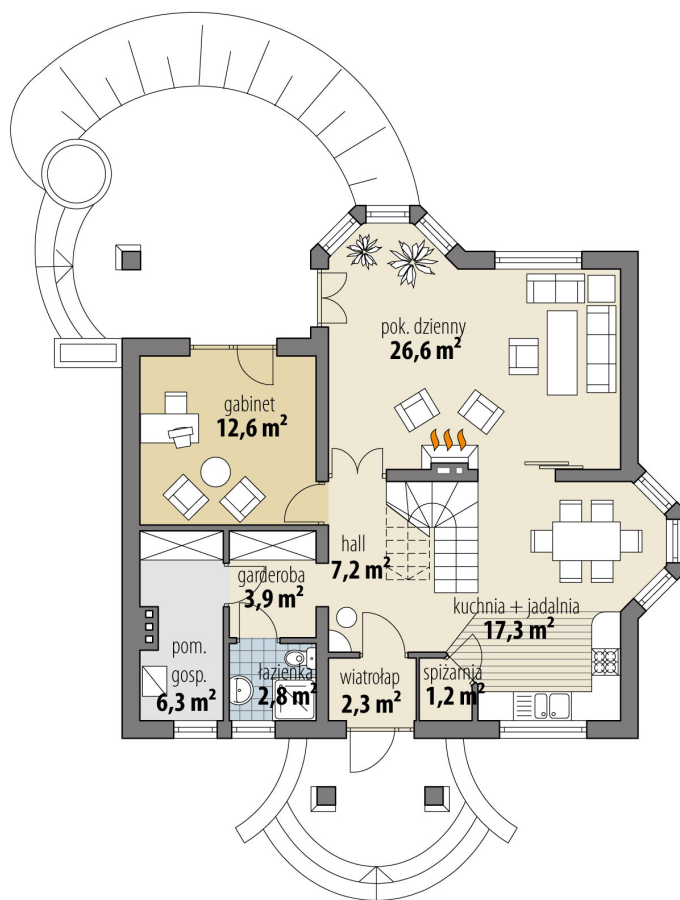
RZUT PARTER
