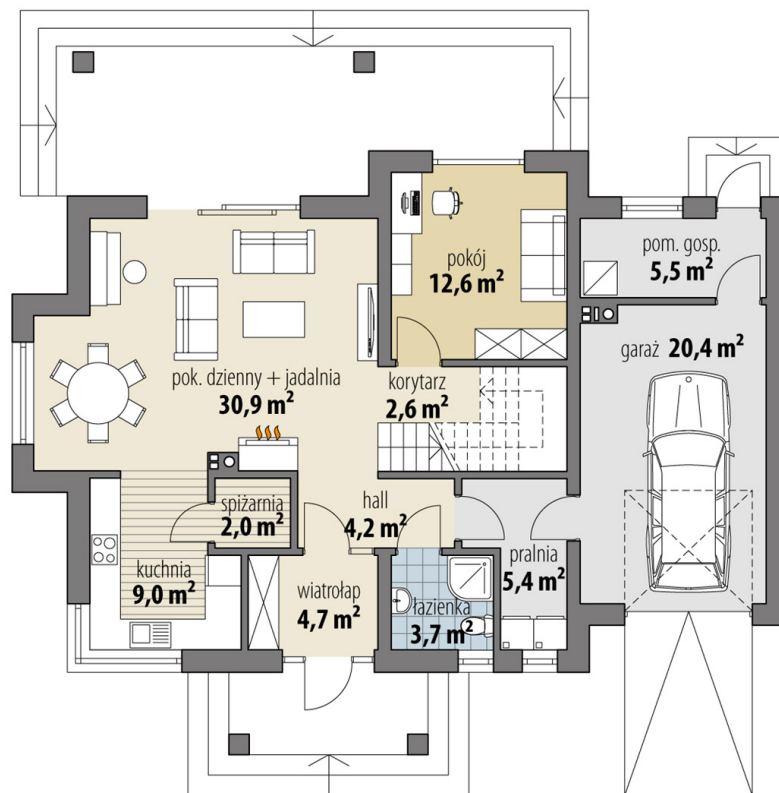
RZUT PARTER
