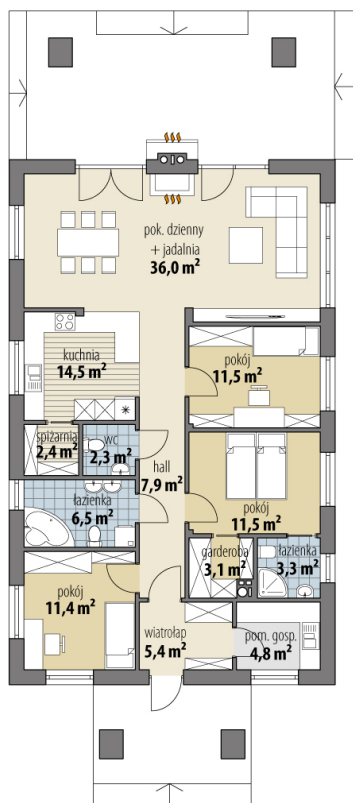
RZUT PARTER
