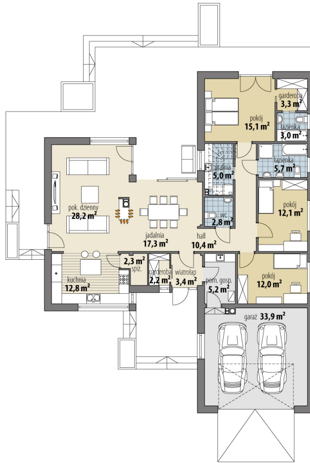
RZUT PARTER
