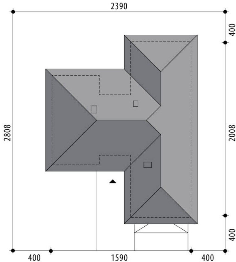
RZUT DZIAŁKI
