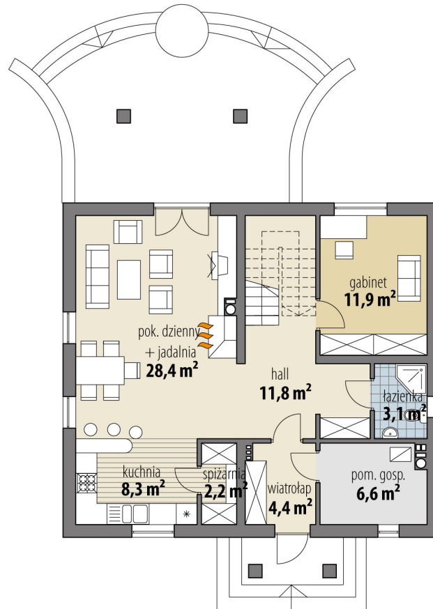
RZUT PARTER
