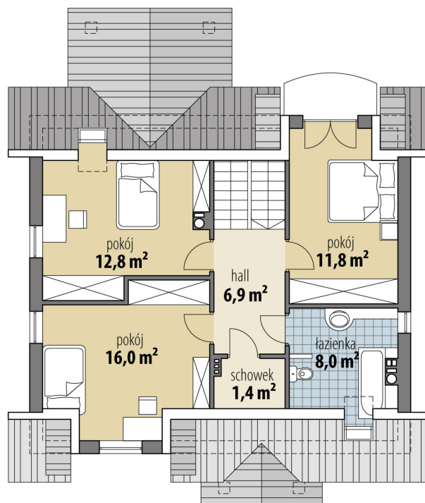
RZUT
