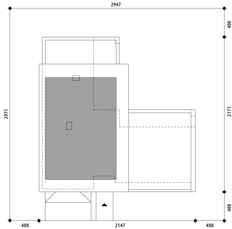
RZUT DZIAŁKI
