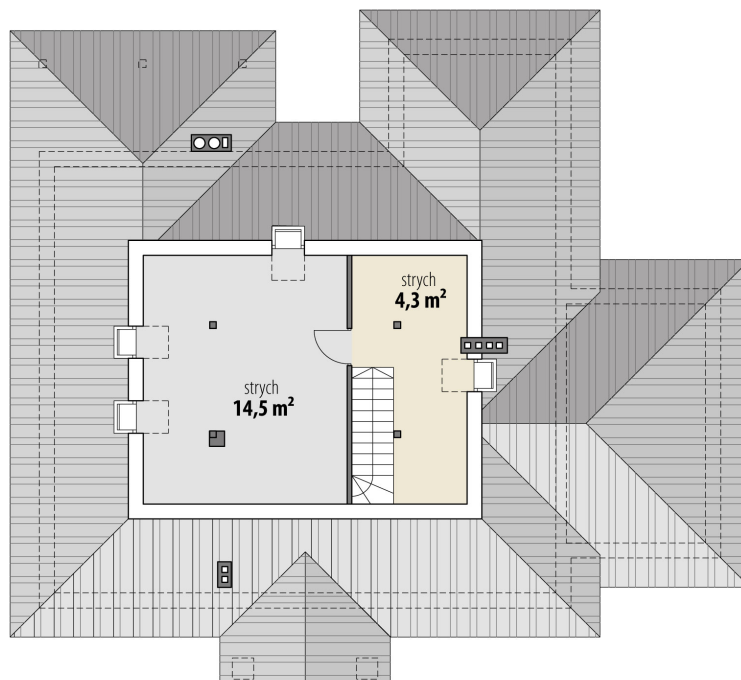
RZUT
