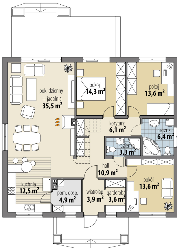
RZUT PARTER
