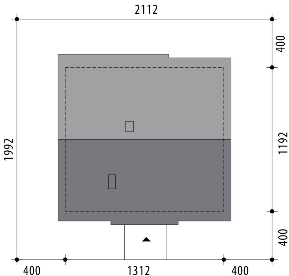
RZUT DZIAŁKI
