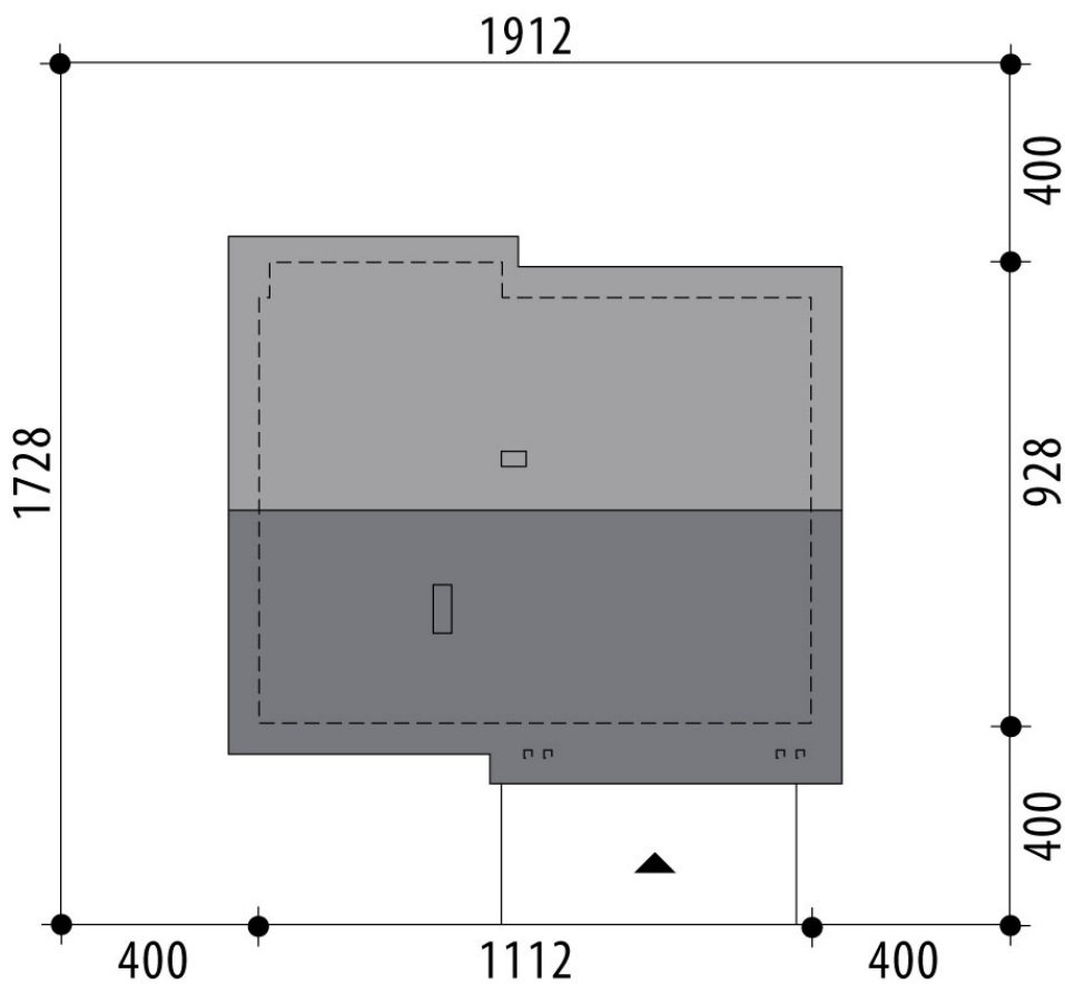
RZUT DZIAŁKI
