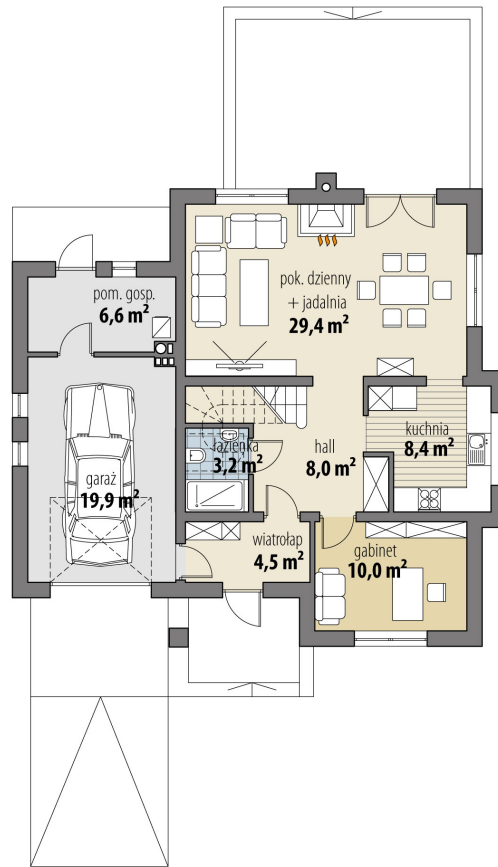
RZUT PARTER
