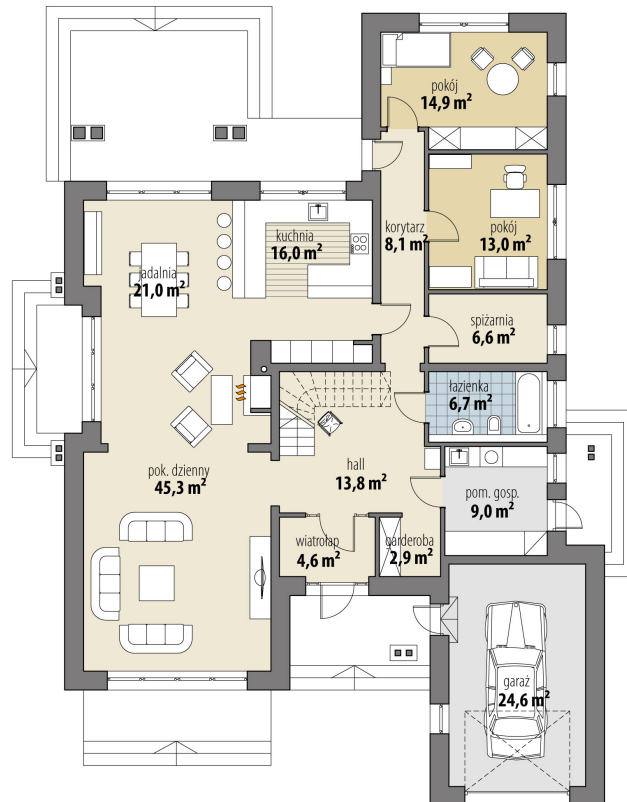
RZUT PARTER
