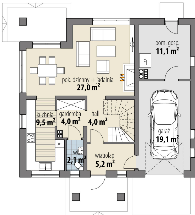
RZUT PARTER
