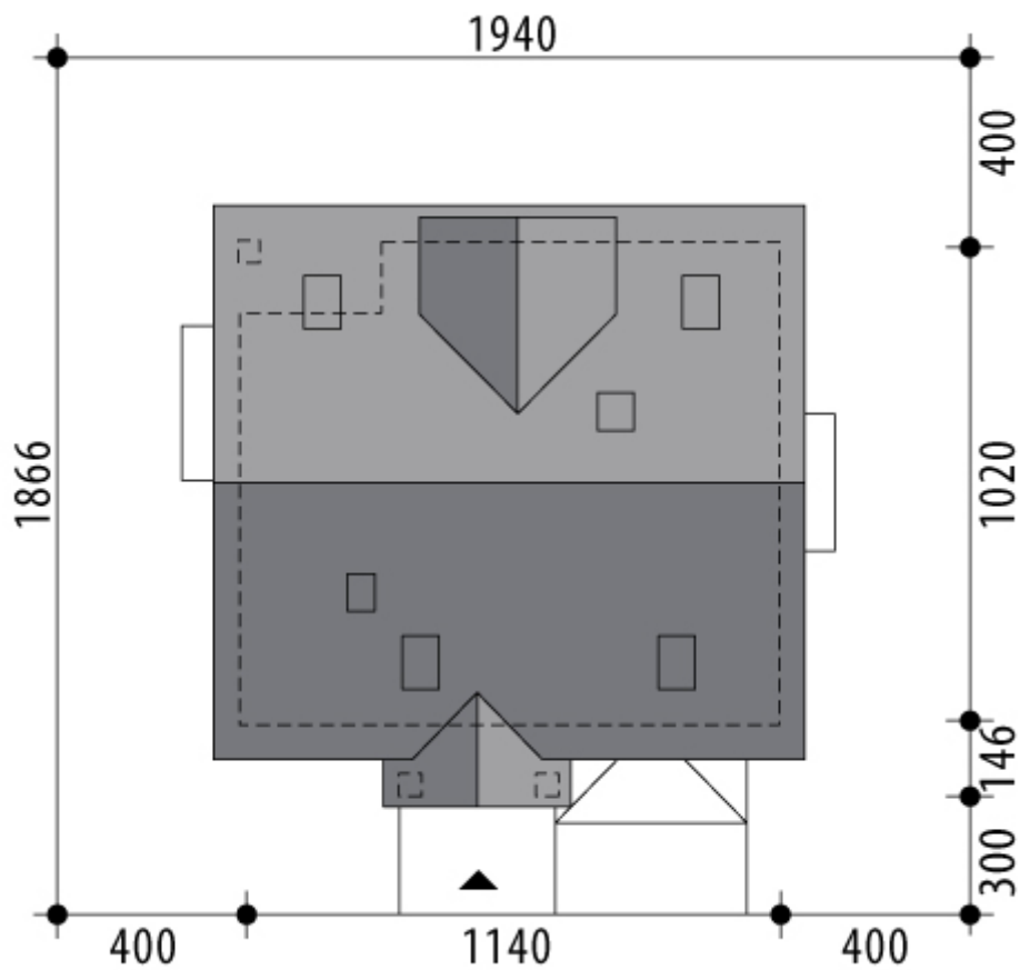
RZUT DZIAŁKI
