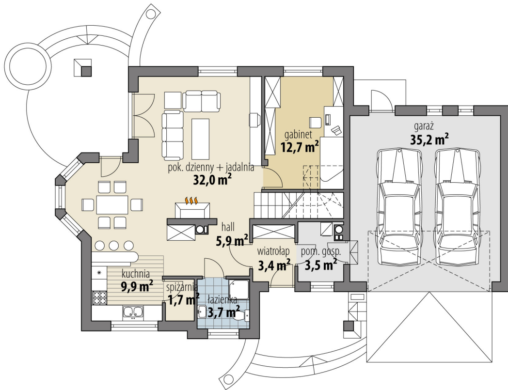
RZUT PARTER
