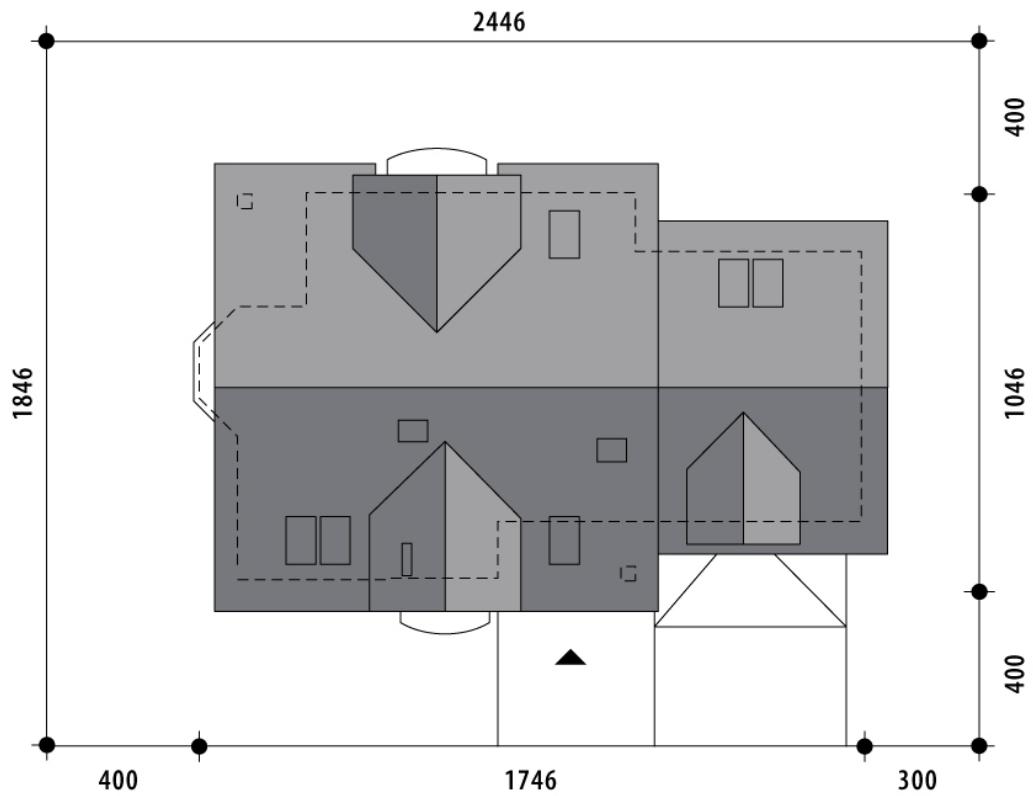
RZUT DZIAŁKI
