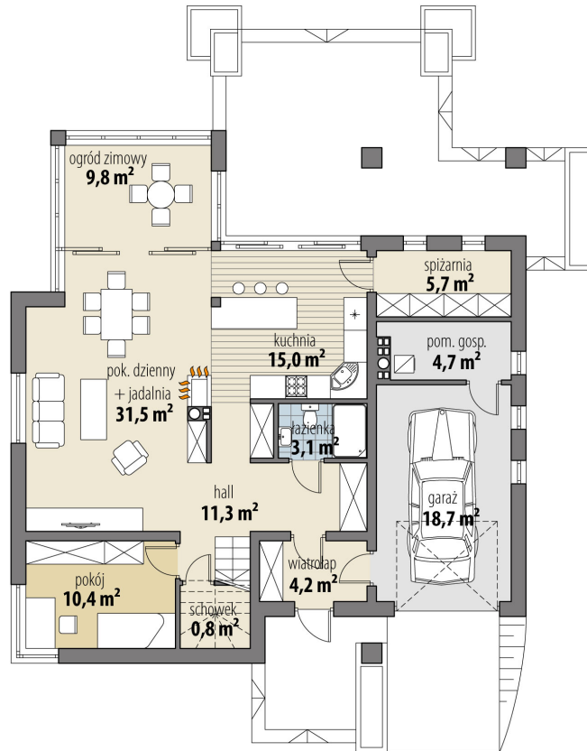
RZUT PARTER
