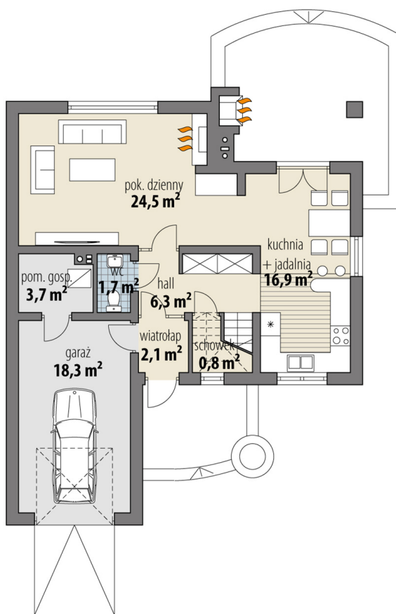
RZUT PARTER
