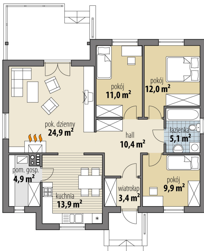
RZUT PARTER
