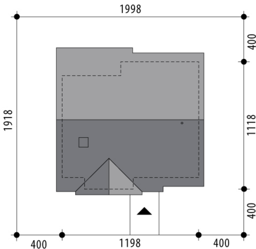
RZUT DZIAŁKI
