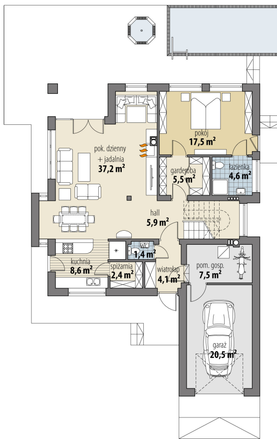
RZUT PARTER
