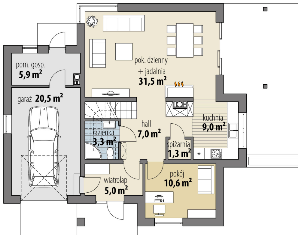
RZUT PARTER
