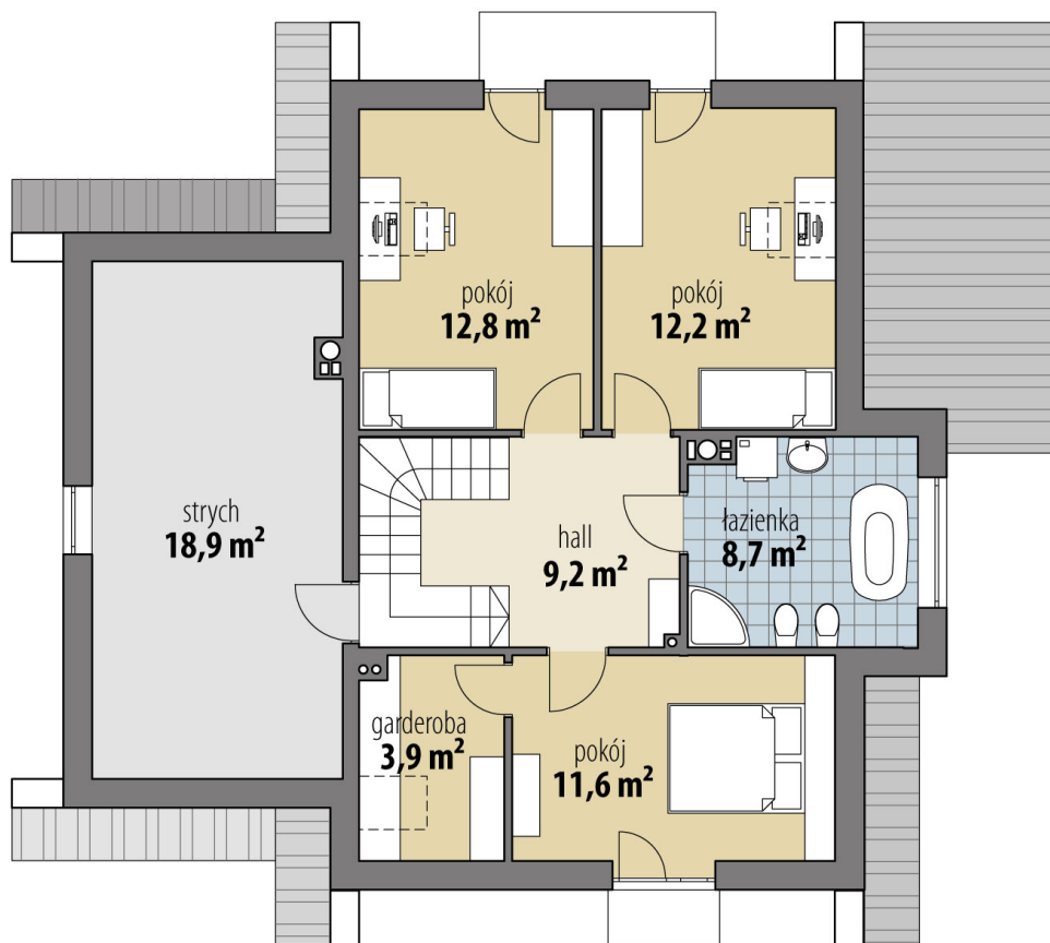
RZUT
