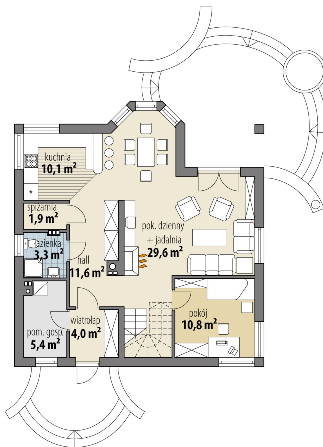
RZUT PARTER
