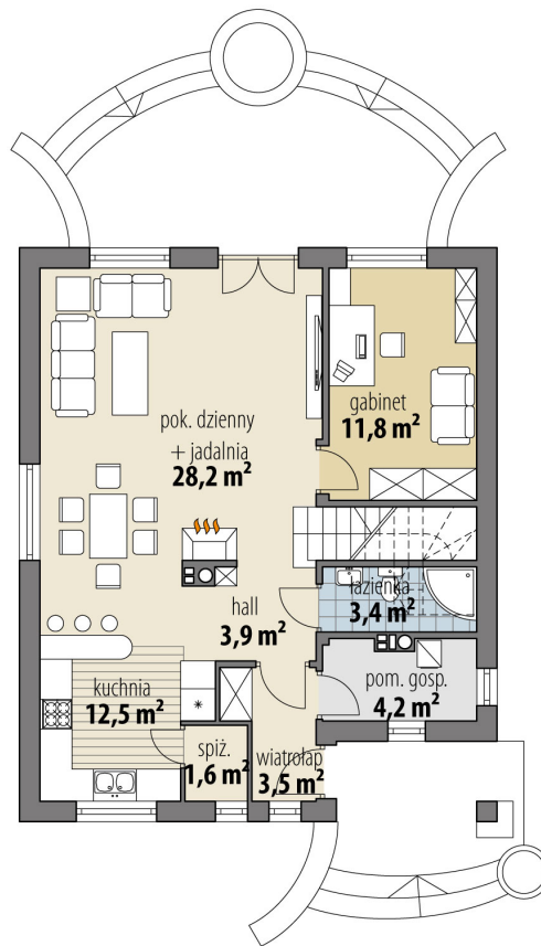
RZUT PARTER
