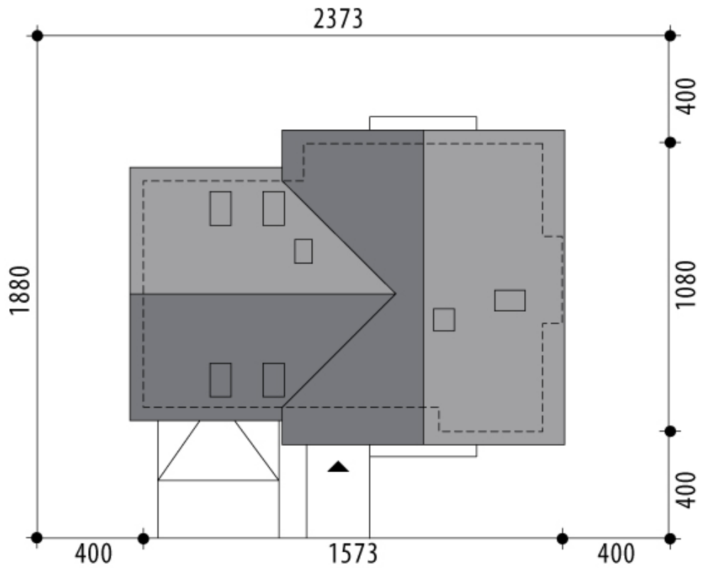
RZUT DZIAŁKI
