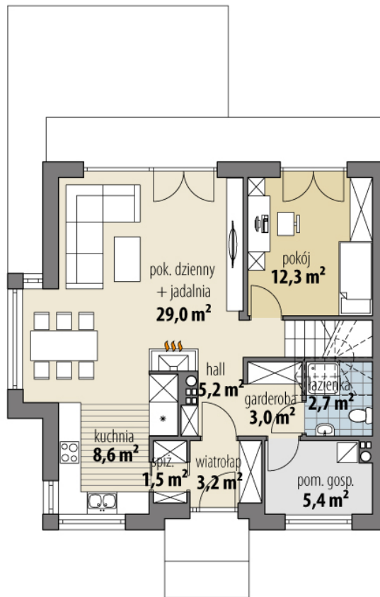
RZUT PARTER
