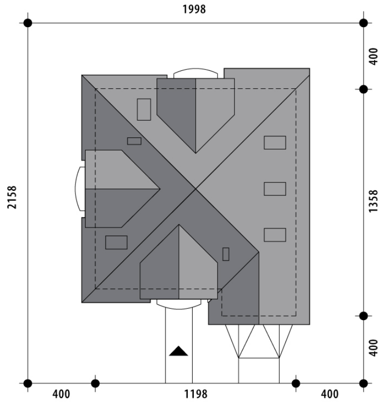
RZUT DZIAŁKI
