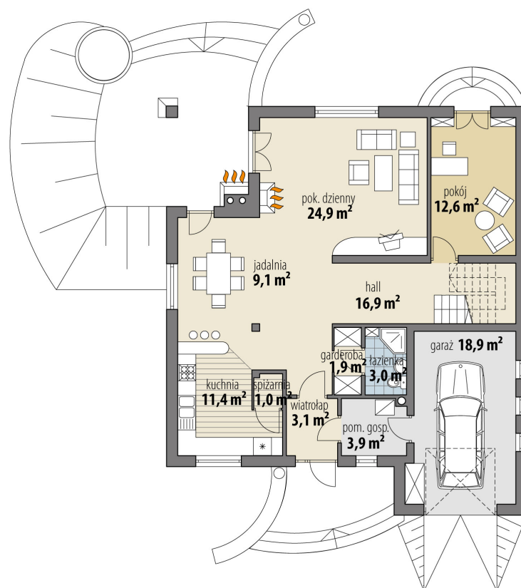
RZUT PARTER
