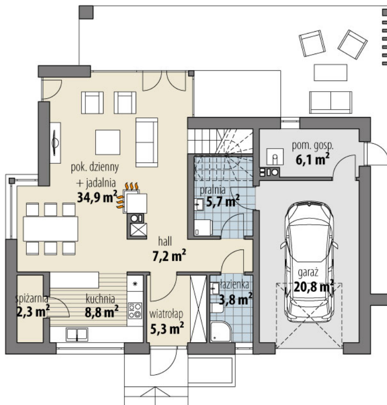
RZUT PARTER
