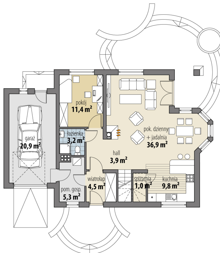
RZUT PARTER
