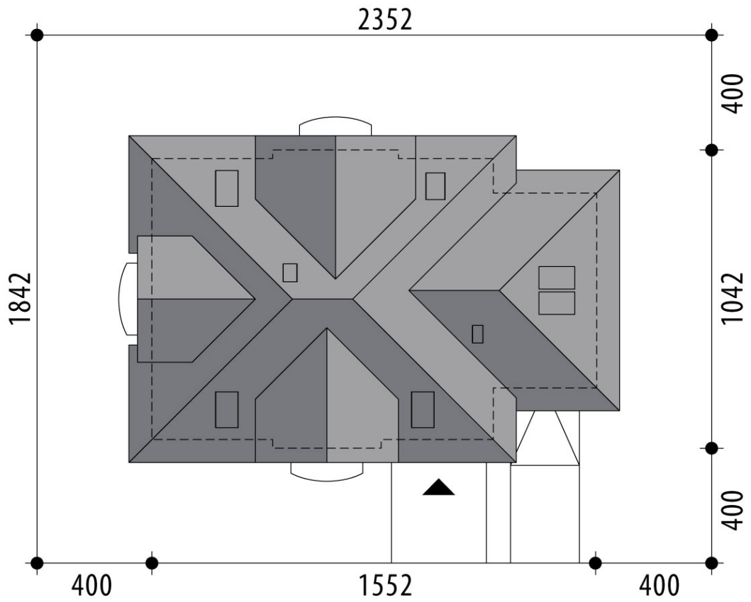
RZUT DZIAŁKI
